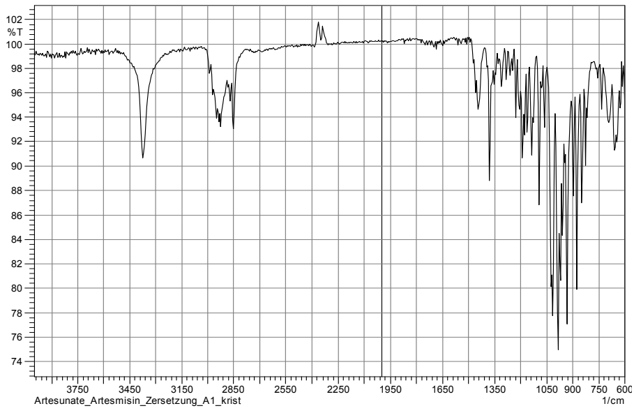
Dihydroartemisinin, Artenimol (3)
