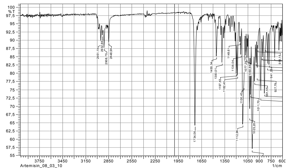
Artemisinin (2)
