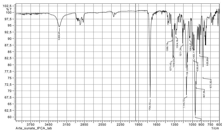
Artesunate (1)
